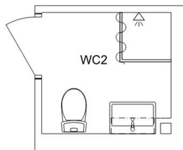
PLAN 1:20
